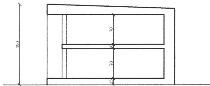
SEZIONE LONGITUDINALE
