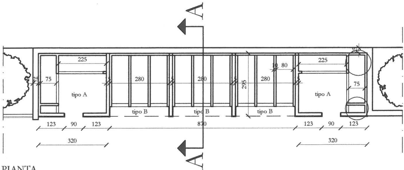
PIANTA
