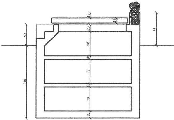
SEZIONE
